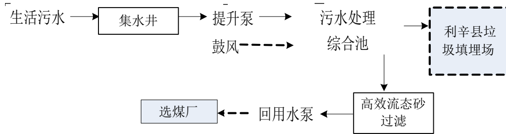
图 7-1 生活污水处理站处理工艺流程图
