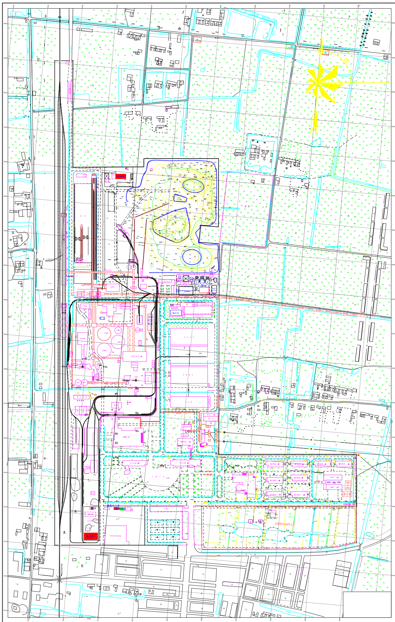
图3-4 板集煤矿工业场地平面布置图
