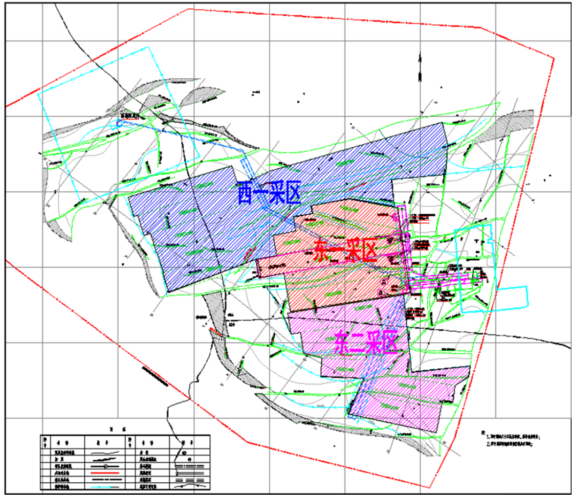
图 3-3 板集矿井采区划分图
