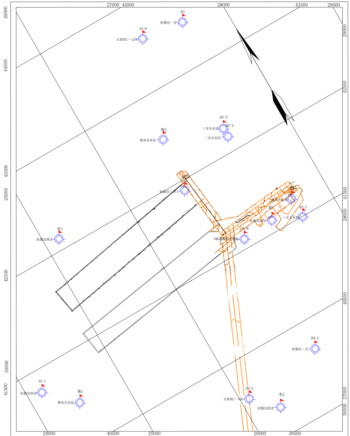
图 6-1 板集煤矿水文长观孔平面分布图
