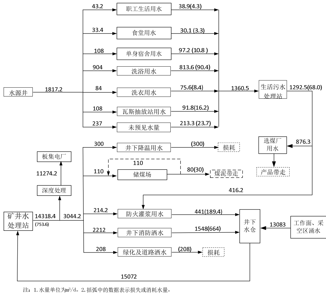
图 3-8 板集煤矿及选煤厂环评阶段水量平衡图
